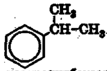
изопропилбензол
