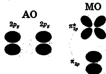
Рис. 3.11. Образование молекулярных \pi -орбиталей из атомных p-орбиталей.
