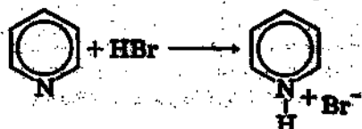
пиридин
