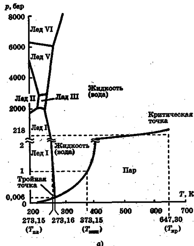
Рис. 3.12. Фазовые диаграммы: а — вода.
