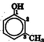
3-метилфенол м-крезол
