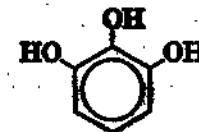
резорцин
