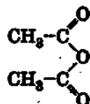
уксусный ангидрид
