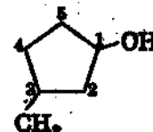
3-метилциклопентанол
