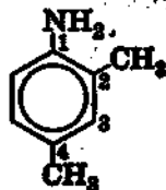
2,4-диметилаанилин
