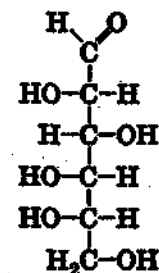
L-глюкоза
