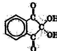
нингидрин
