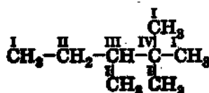
Разветвленный скелет
