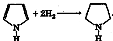
пирролидин
