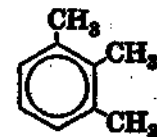
1,2,3-триметилбензол
