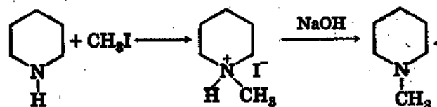
N-метилпиперидин
