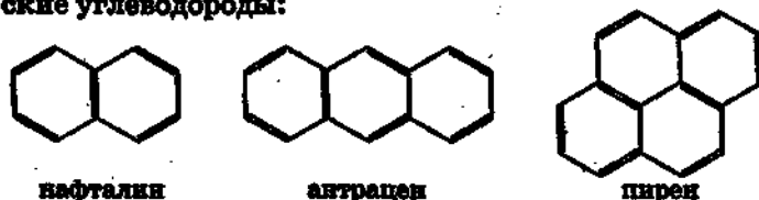
нафталин
