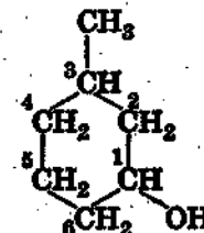
3-метилциклогексано́л
