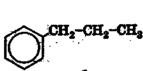
пропилбензол
