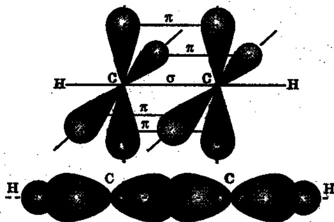
Рис. 3.8. Образование \sigma - и \pi -связей в молекуле C_2H_4 .
