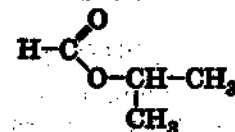
изопропилформиат
