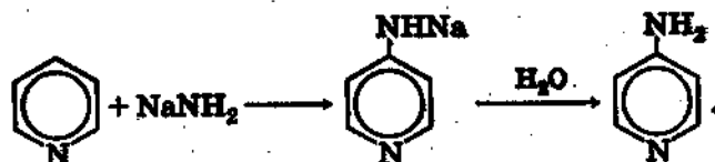
л-аминопиридин
