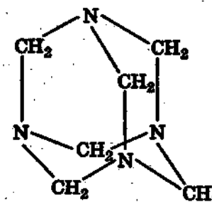
гексаметиленetetрамин (уротропин)
